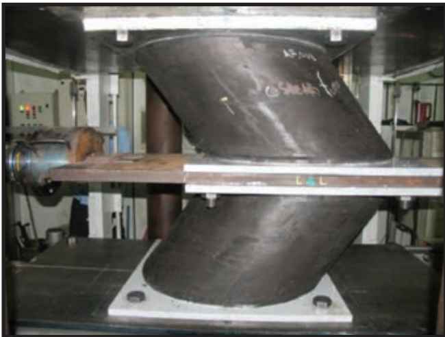
Kauçuk Esaslı Sismik İzolatör
