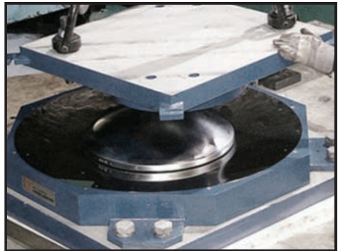
Sürtünme Esaslı Sarkaç Tipi Sismik İzolatör
